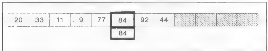
Bild 1. Schematische Darstellung eines Files mit Filepuffer
